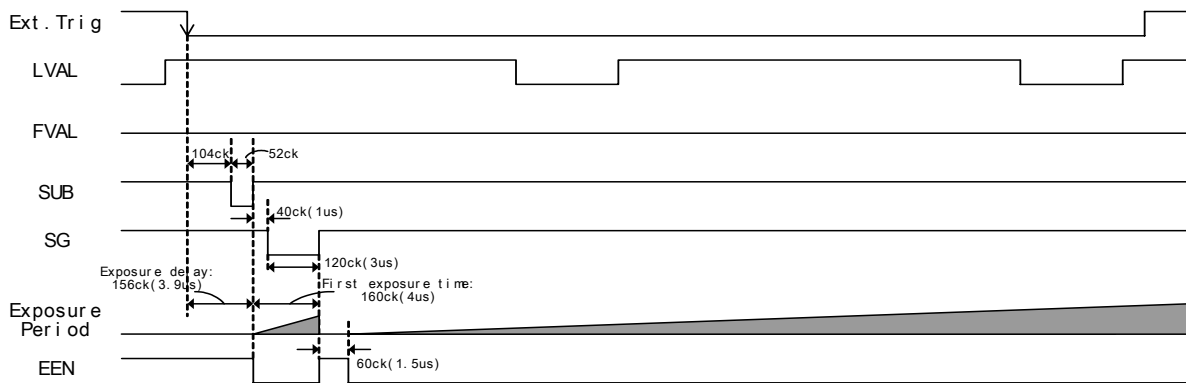
Fig. 28A. PIV mode details
